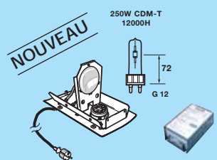
⑬ CDM-T 250W Froid G12
