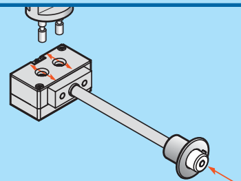
⑨ Douille G22 série 700 SX2.
